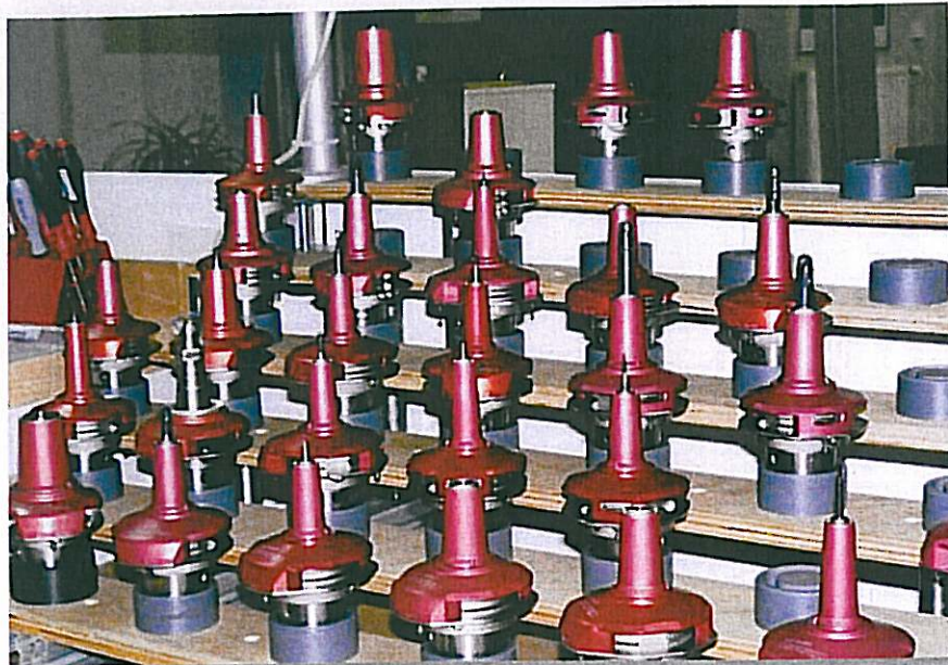
Bild 1: Den Medium-Verteiler gibt es in den Größen HSK 25, HSK 32, HSK 40, HSK 50 und HSK 63, für Werkzeuge von 0,2 mm bis 38 er Messerkopf. Auf Wunsch sind aber auch andere Größen lieferbar
