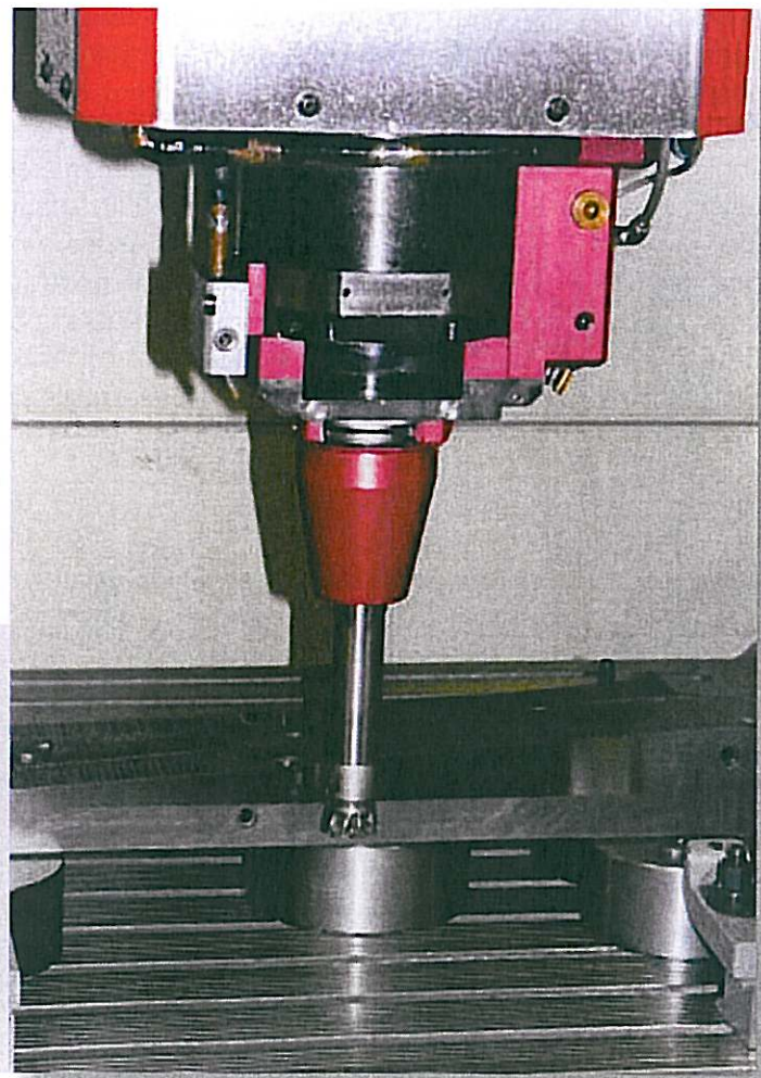
Bild 5: Selbst bei weniger anspruchsvollen Bauteilen sind damit mit dem Medium-Verteiler eine höhere Prozesssicherheit und Standzeitverlängerung der Werkzeuge zu erzielen
